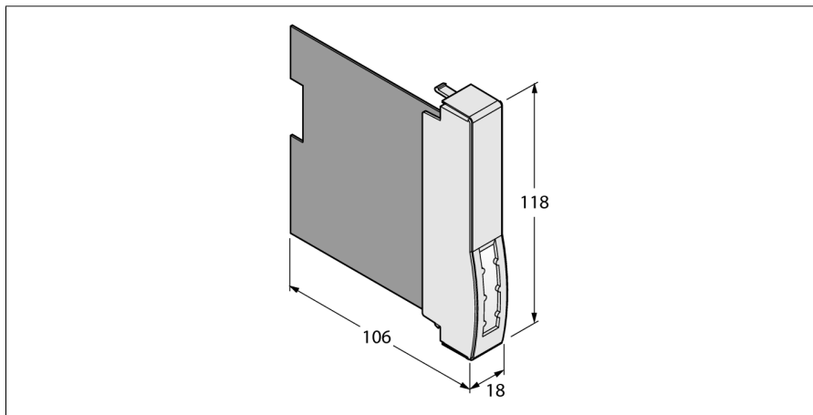
■ Модуль-заглушка для неиспользованных слотов в стойке
